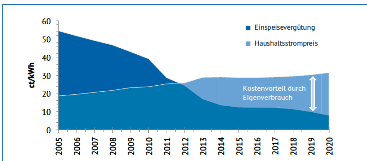
Entwicklung von Einspeisevergütung und Haushaltsstrompreis zwischen 2005 und 2020
